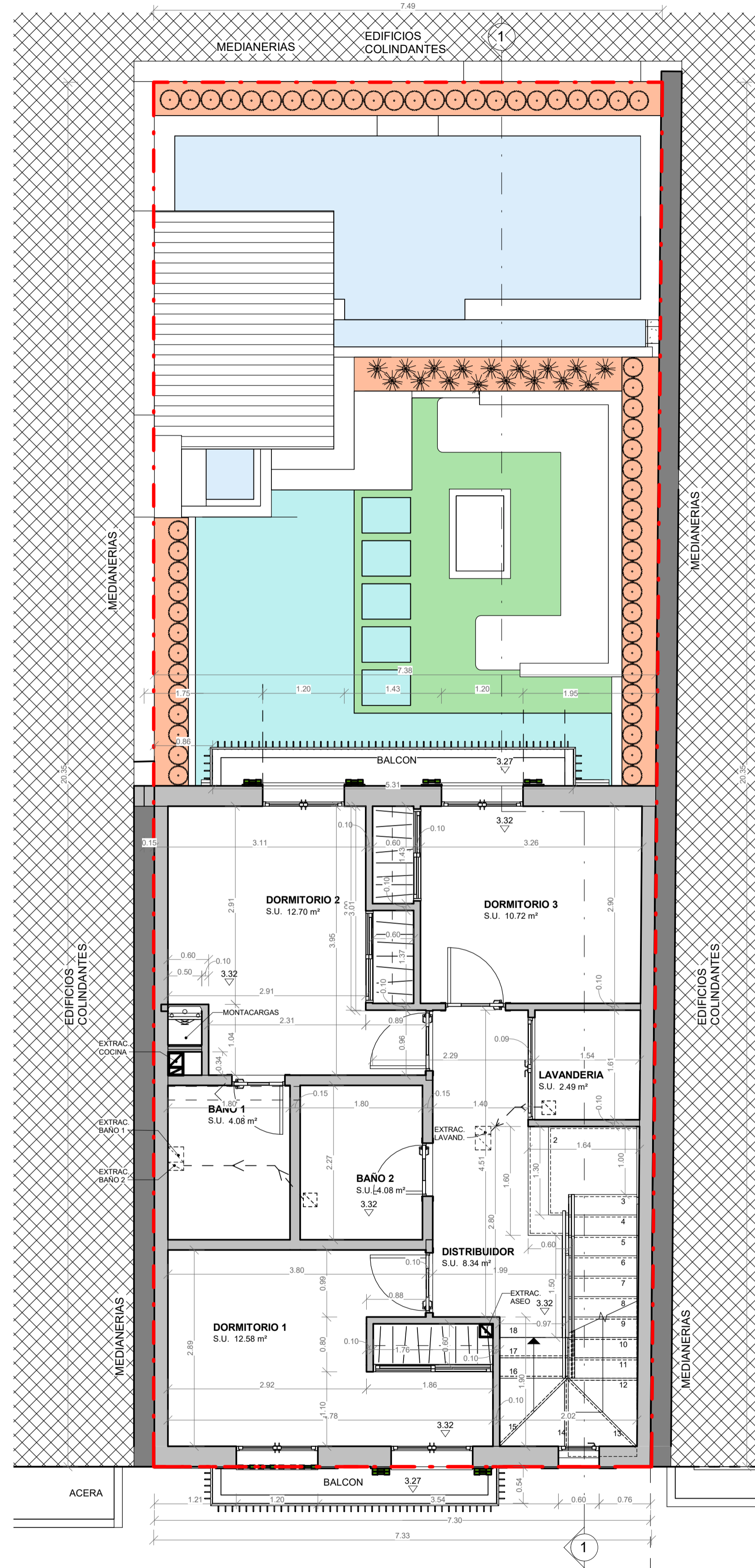
2 04 PLANTA PISO 1° ACOTADA 5 1 : 50
