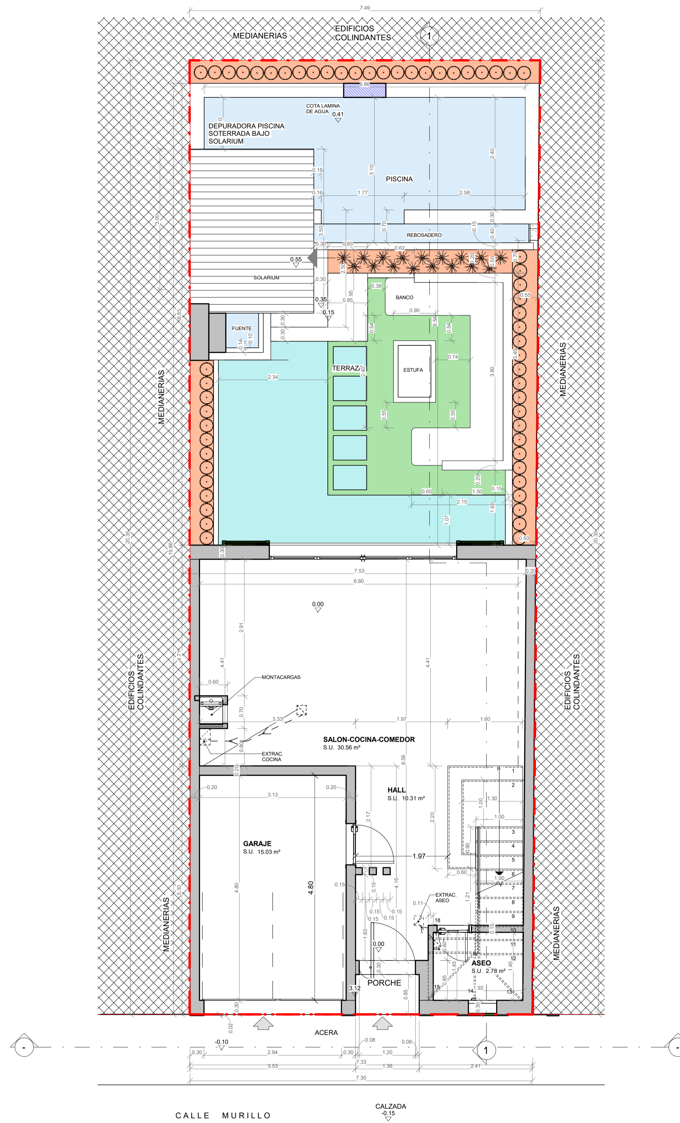
2 05 PLANTA BAJA ACOTADA 4 1:50
