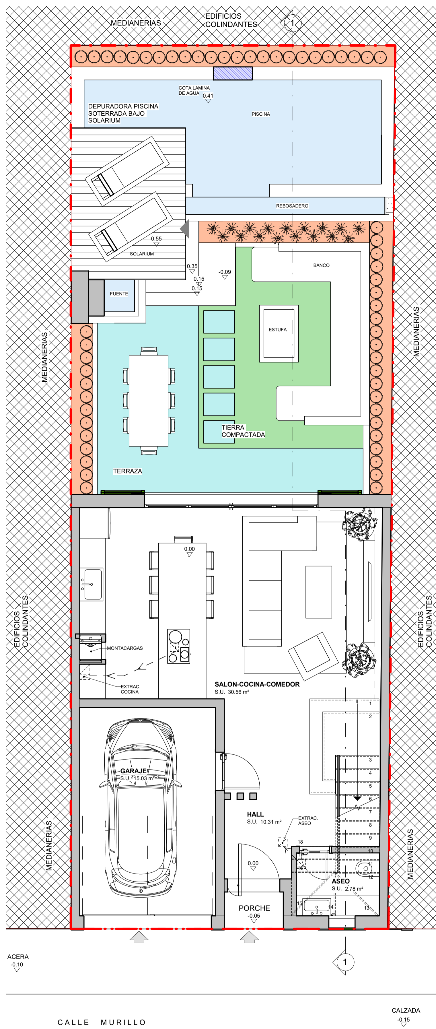
1 05 PLANTA BAJA 4 1:50
